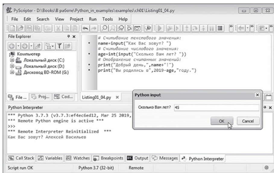
Рис. 1.39. Ввод возраста в поле ввода диалогового окна
