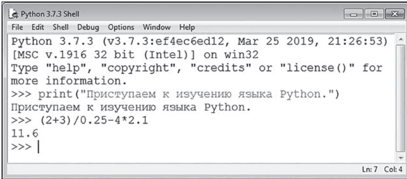
Рис. 1.4. Результат вычисления арифметического выражения
