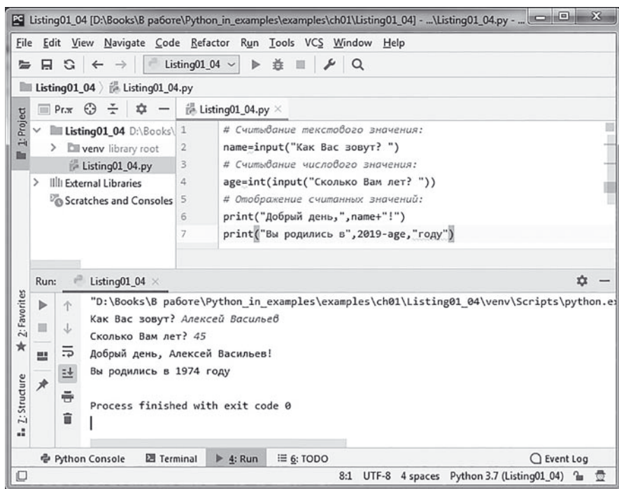
Рис. 1.36. Результат выполнения программы в окне среды разработки PyCharm
