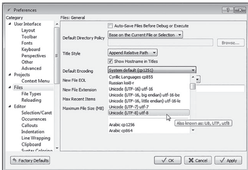
Рис. 1.26. Выбор используемой по умолчанию кодировки для файлов с программным кодом
