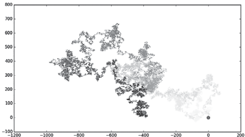
Рис. 15.11. Случайное блуждание с 50 000 точек
